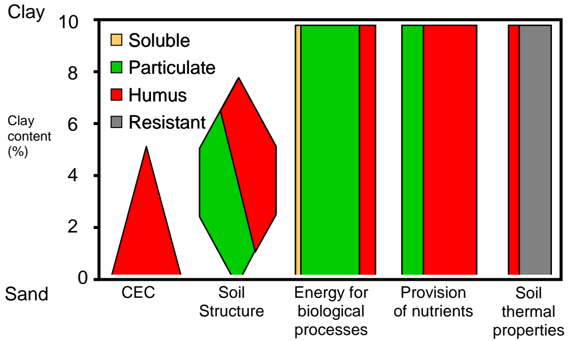
Figure 4: Proposed importance of SOM composition in determining SOM function
